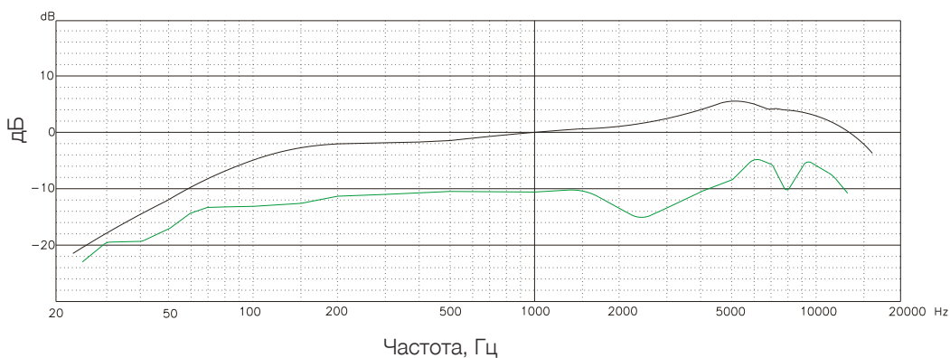
Частотный диапазон
