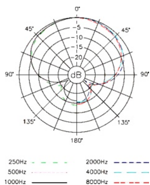
Диаграмма направленности
